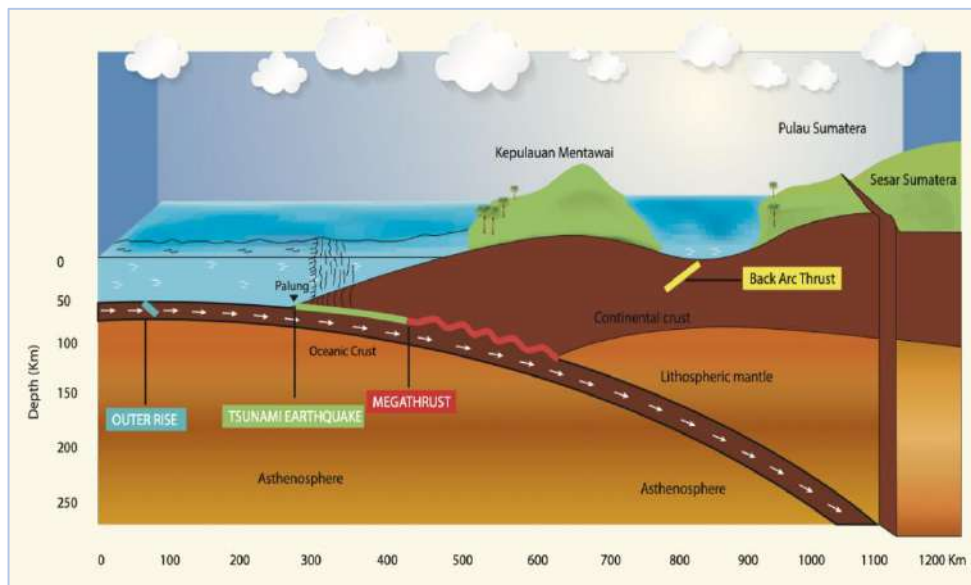
Gambar 2.17 Proses terjadinya gempa bumi tektonik
